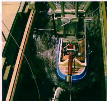
Beproeving van een model van een Lemmeraak in ondiep water in de sleeptank van de TU Delft.
