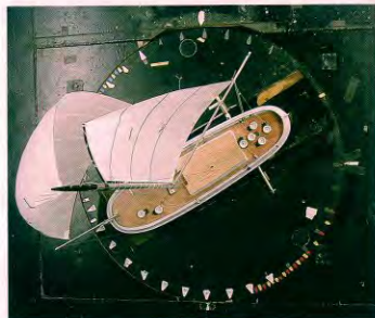
Beproeving van een model van een Lemmeraak in de windtunnel van de University van Southampton.
